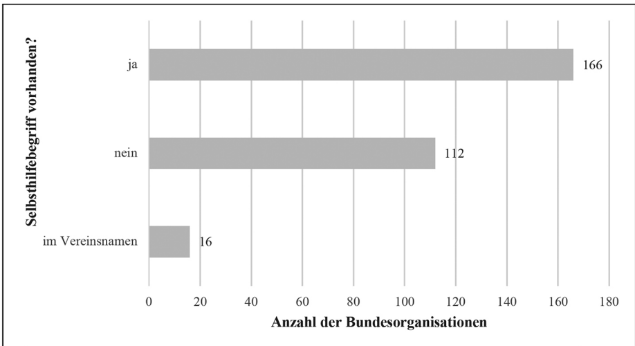
Abb. 3: Häufigkeitsanalyse
