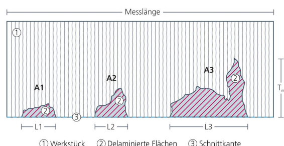
Bild 2 Kenngrößen zur Bewertung der Schnittqualität an der Werkstückkante auf Basis der delaminierten Fläche (A1, A2, A3) sowie der maximalen Tiefe der Delamination. Grafik: [10]
